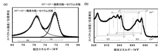
白金担持量が0.5wt%の電極を構成するセリアナノワイヤと白金との界面のXPS測定結果
